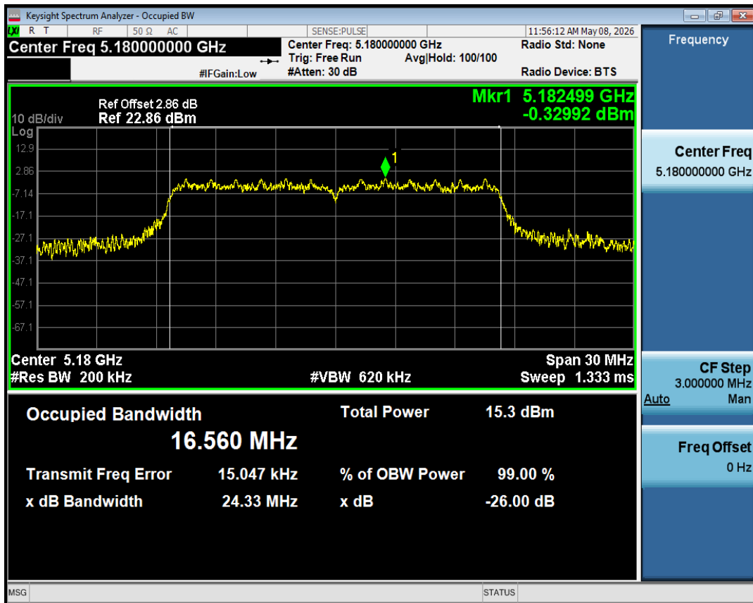
OBW NVNT a 5180MHz Ant1
