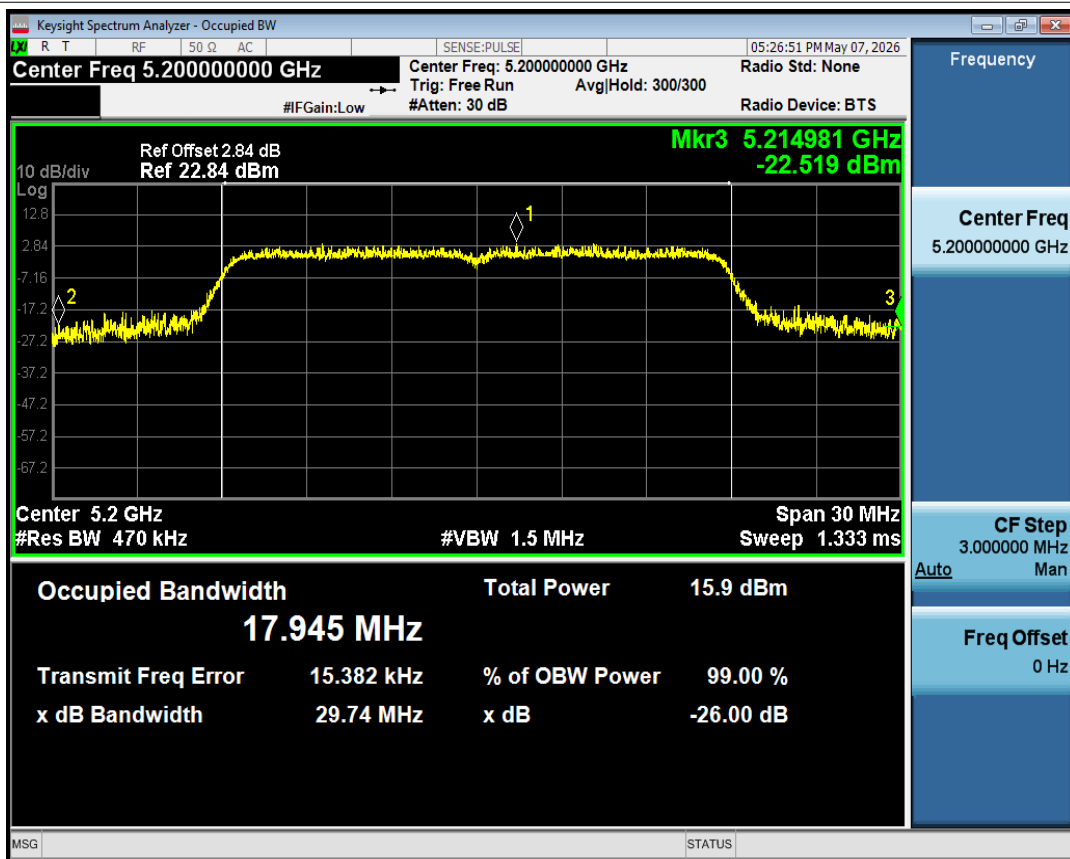
-26dB Bandwidth NVNT ac20 5200MHz Ant1
