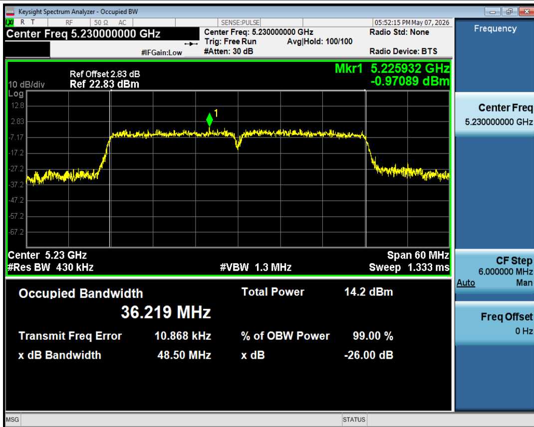
OBW NVNT ax40 5230MHz Ant1
