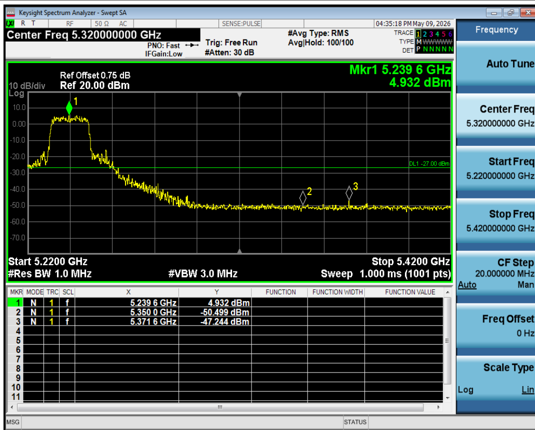
Band Edge NVNT ax20 5240MHz High Ant1
