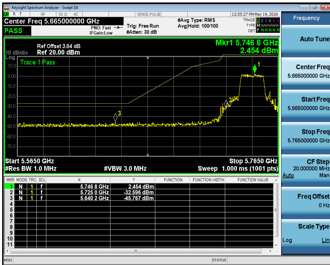
Band Edge NVNT ax20 5745MHz Low Ant1
