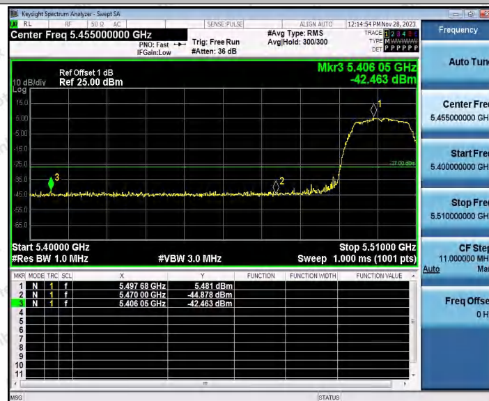
11A_Ant1_Low_5500
