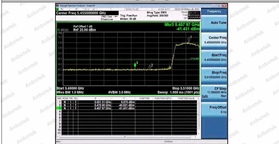
11AX20SISO_Ant1_Low_5500
