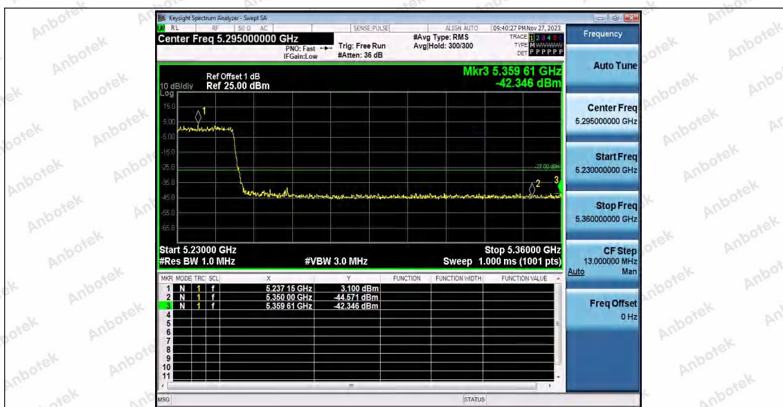
11AX40SISO_Ant1_Low_5270
