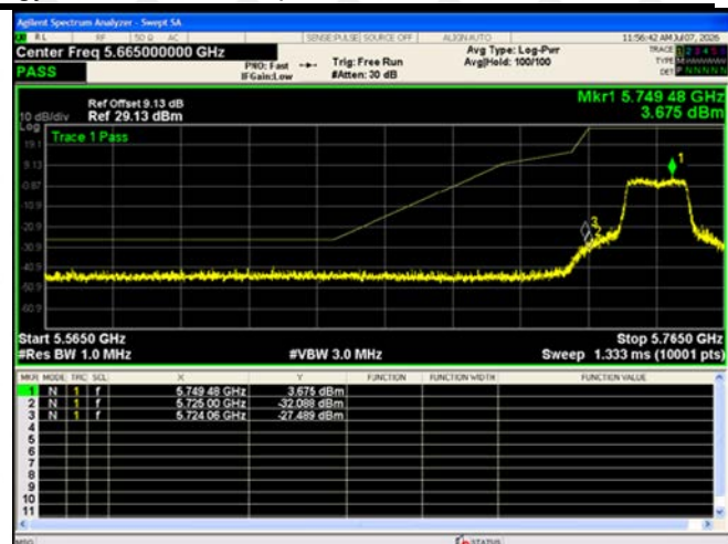
802.11(n40)-5755
