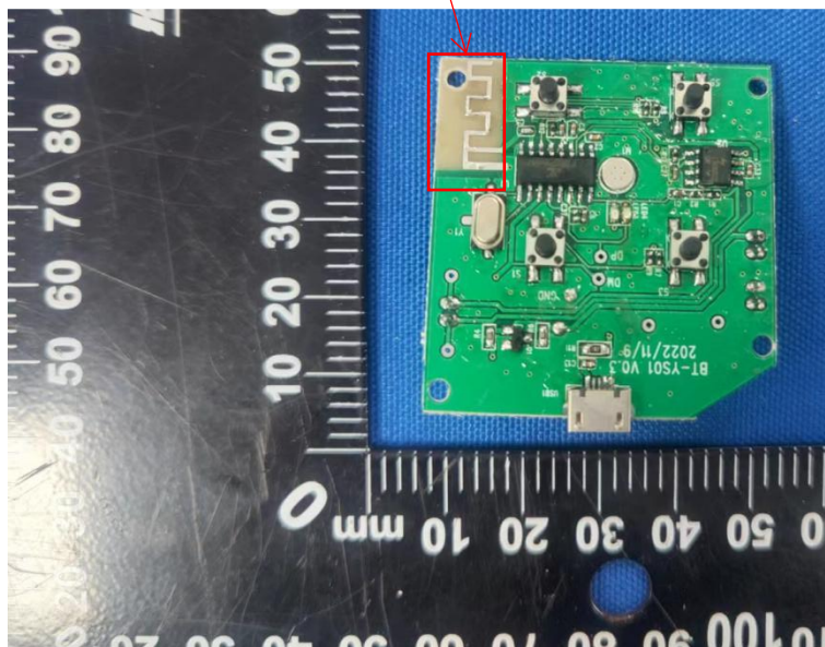
Antenna
