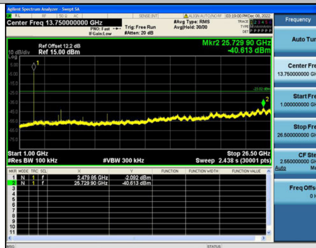
3DH5-Ant1-2480-0-Reference-5.51
