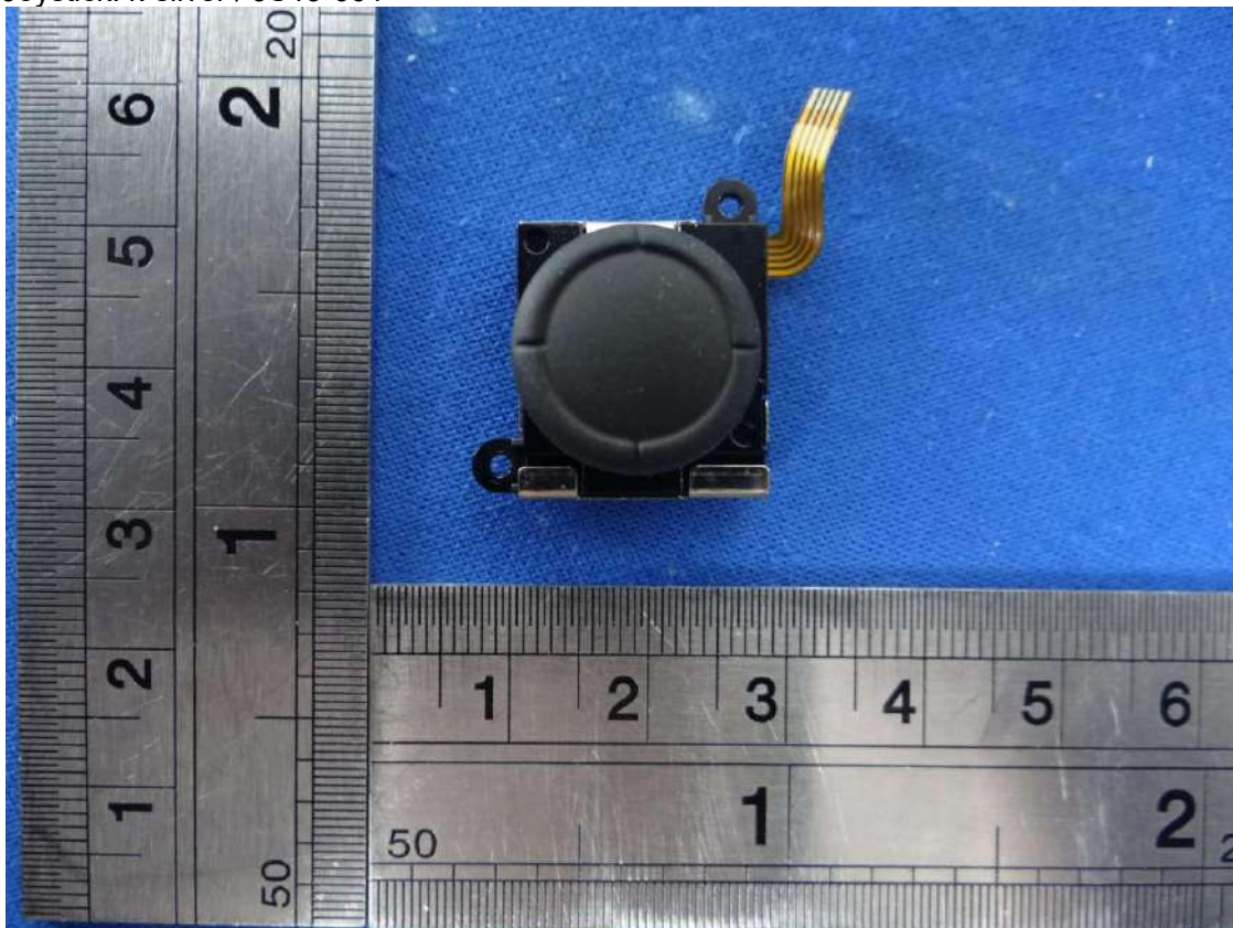
Joystick: k-silver / JS19-001
