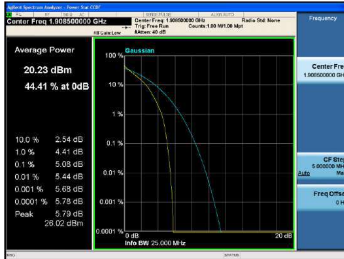
Band2-3MHz-QPSK-19185-15RB#0
