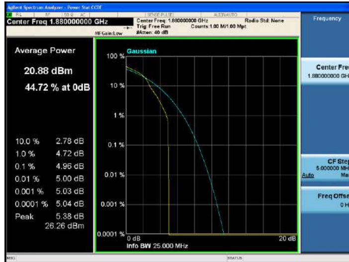
Band2-20MHz-16QAM-18900-1RB#0
