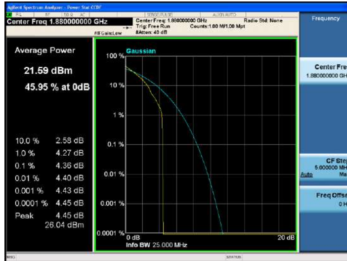
Band2-10MHz-QPSK-18900-1RB#0
