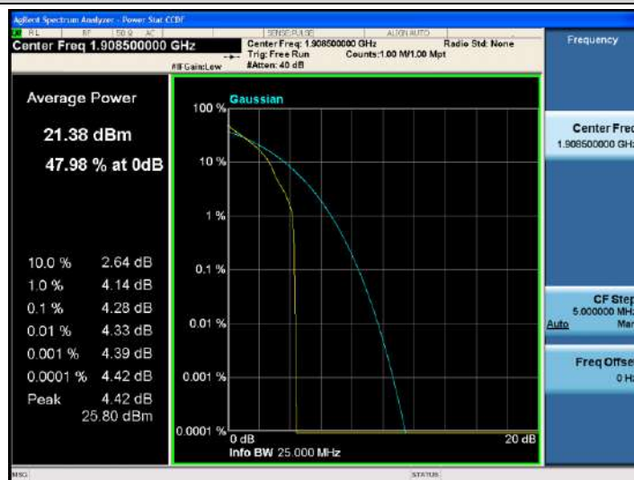
Band2-3MHz-QPSK-19185-1RB#0
