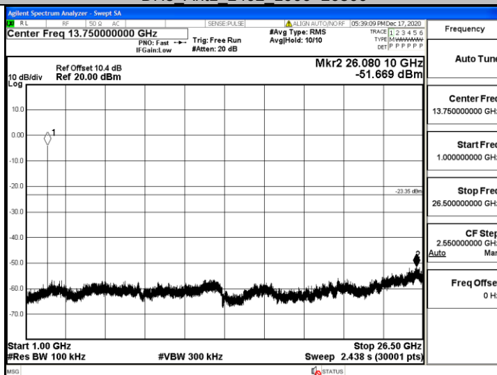
DH5_Ant1_2402_1000~26500
