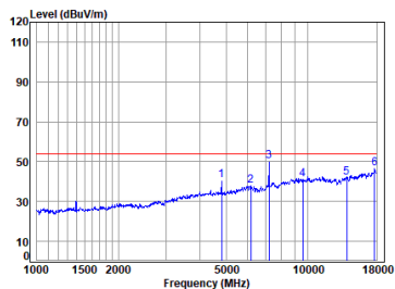
BLE_2M_TX_CH_01_Horizontal-Avg
