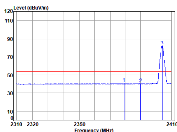
BLE_2M_TX_CH_01_Horizontal-Avg
