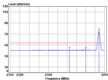
BLE_2M_TX_CH_01_Vertical-Avg
