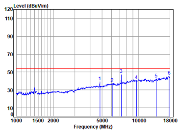
BLE_2M_TX_CH_01_Vertical-Avg
