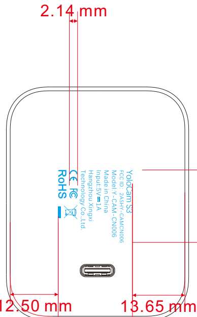
产品主体, 后视图
