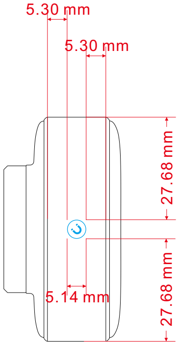
产品主体, 右视图
