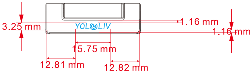
产品支架正面, 正视图
