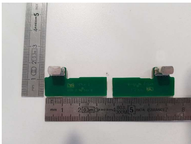
AVW0171 – Wi-Fi antennas
