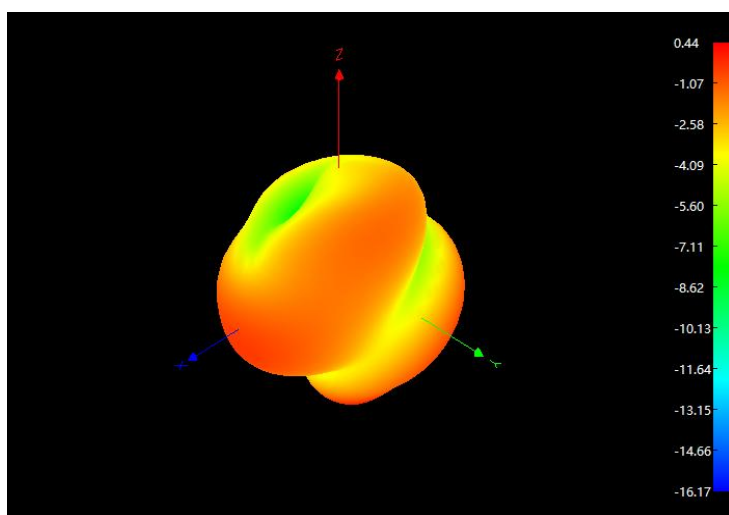
2500MHz 3D
