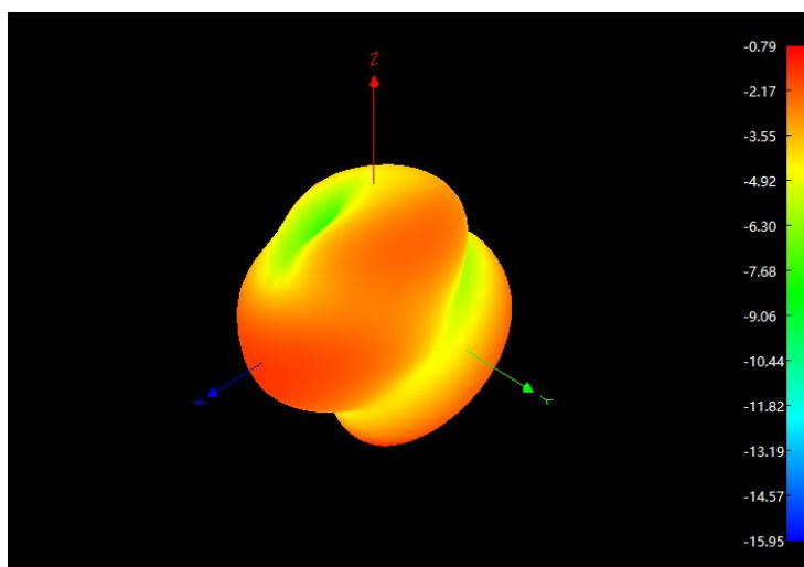
2450MHz 3D
