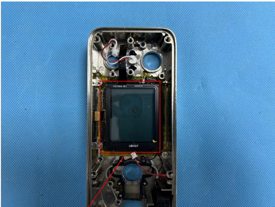
NFC Antenna
