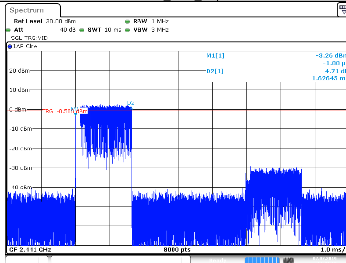
3DH3_Ant0_Hop
