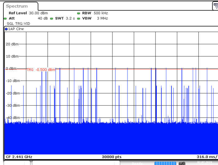
3DH5_Ant0_Hop
