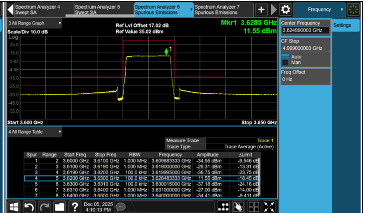
CH 641666 (3624.99 MHz)
