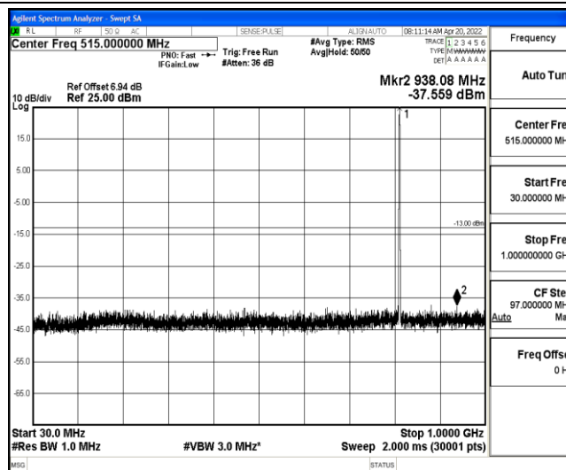
Band26-10MHz-QPSK-26740-1-0-Low-30-1000--37.56-PASS
