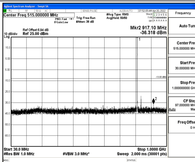
Band26-5MHz-QPSK-26715-1-0-Low-30-1000--36.32-PASS
