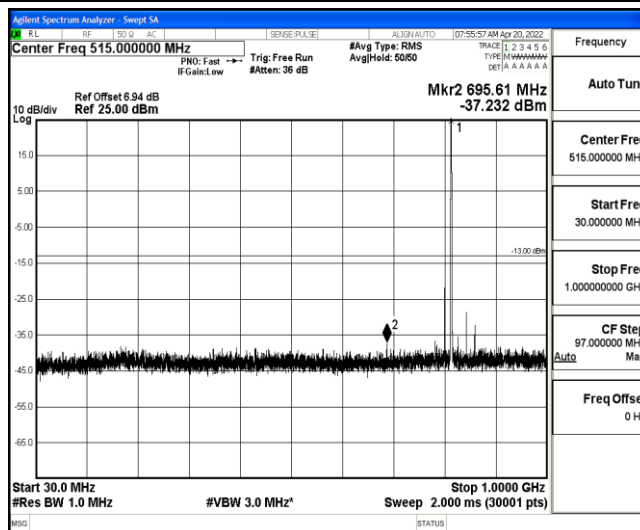
Band26-5MHz-QPSK-26740-1-0-Low-30-1000--37.23-PASS
