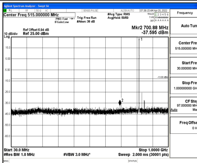
Band26-3MHz-16QAM-26740-1-0-Low-30-1000--37.6-PASS
