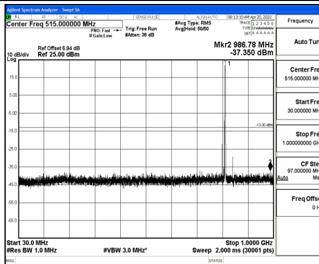
Band26-10MHz-16QAM-26740-1-0-Low-30-1000--37.35-PASS
