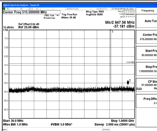
Band26-5MHz-16QAM-26715-1-0-Low-30-1000--37.18-PASS
