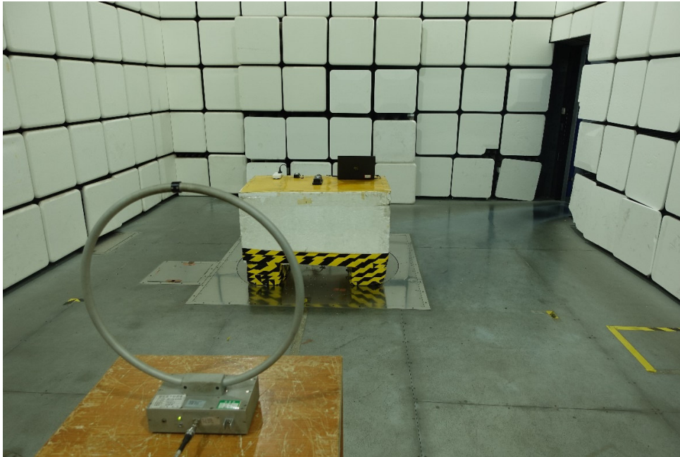
9kHz-30MHz
