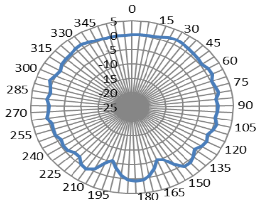
YZ-2450MHz
