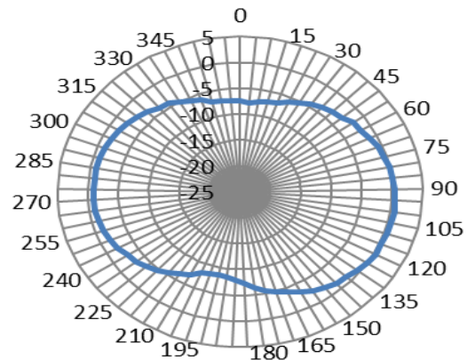
XY-2450MHz
