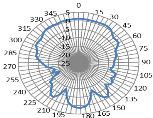
XZ-2450MHz
