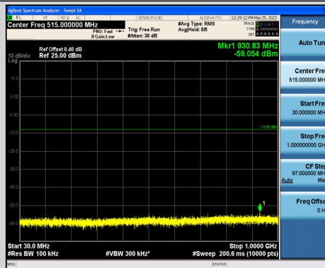
Band4-1.4MHz-QPSK-20175-1-0-Low-30-1000--59.05-PASS
