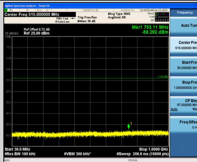
Band2-20MHz-QPSK-18700-1-0-Low-30-1000--59.29-PASS
