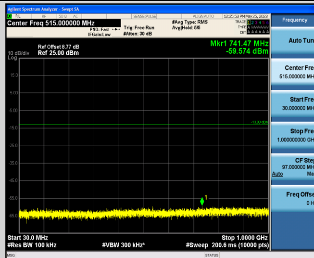
Band4-1.4MHz-16QAM-19957-1-0-Low-30-1000--59.57-PASS
