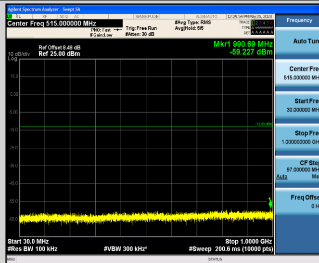
Band4-1.4MHz-QPSK-20393-1-0-Low-30-1000--59.23-PASS
