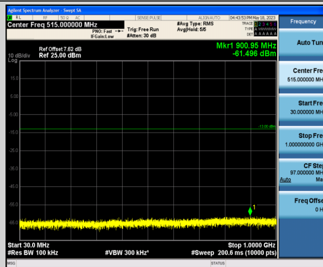
Band2-5MHz-16QAM-18900-1-0-Low-30-1000--61.5-PASS
