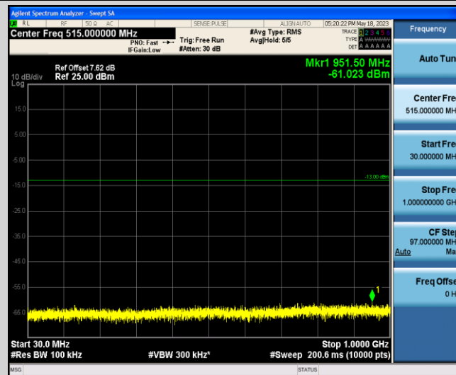
Band2-20MHz-QPSK-18900-1-0-Low-30-1000--61.02-PASS
