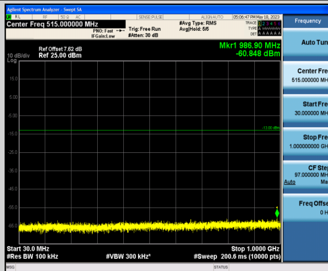
Band2-10MHz-QPSK-18900-1-0-Low-30-1000--60.85-PASS
