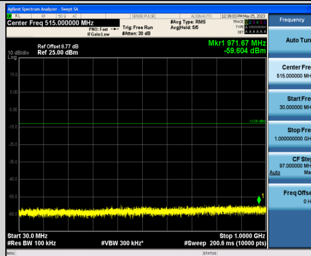
Band4-3MHz-QPSK-19965-1-0-Low-30-1000--59.6-PASS
