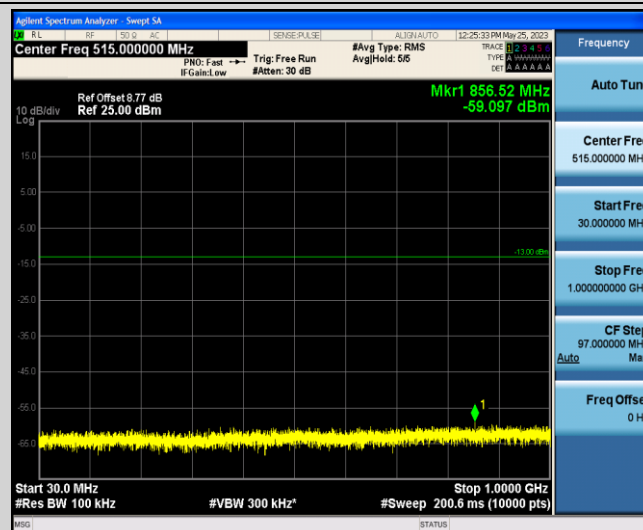
Band4-1.4MHz-QPSK-19957-1-0-Low-30-1000--59.1-PASS
