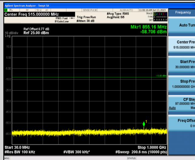
Band4-20MHz-16QAM-20050-1-0-Low-30-1000--58.71-PASS
