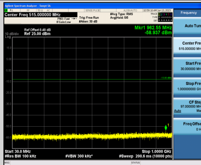
Band4-5MHz-QPSK-20375-1-0-Low-30-1000--58.94-PASS
