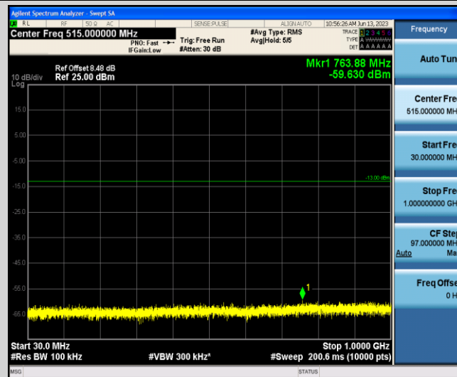
Band4-3MHz-QPSK-20385-1-0-Low-30-1000--59.63-PASS
