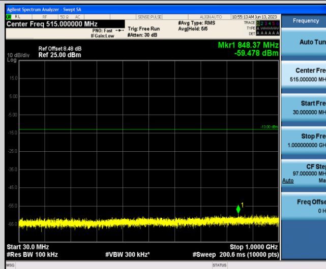
Band4-3MHz-QPSK-20175-1-0-Low-30-1000--59.48-PASS
