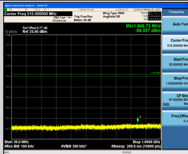
Band4-10MHz-QPSK-20000-1-0-Low-30-1000--59.06-PASS
