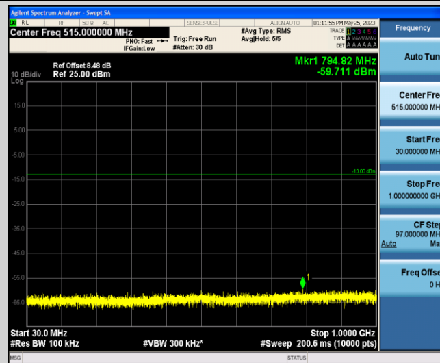
Band4-15MHz-QPSK-20325-1-0-Low-30-1000--59.71-PASS
