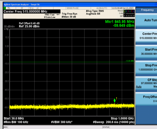
Band4-10MHz-16QAM-20350-1-0-Low-30-1000--59.65-PASS
