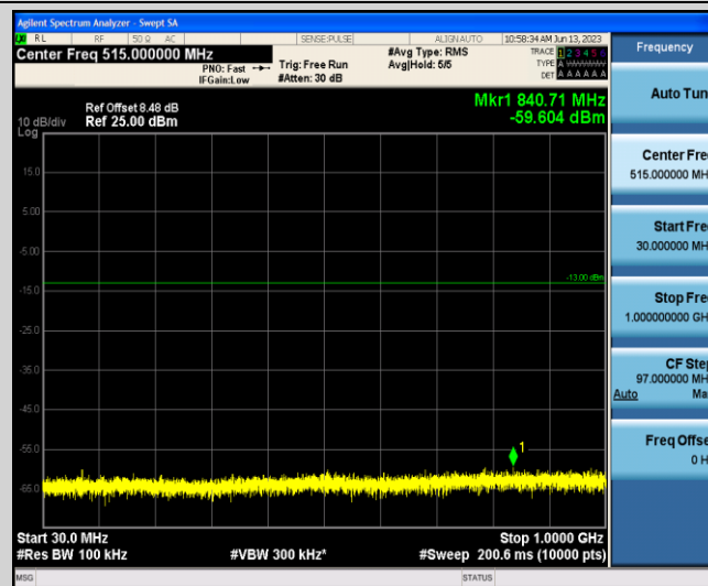
Band4-5MHz-QPSK-20175-1-0-Low-30-1000--59.6-PASS
