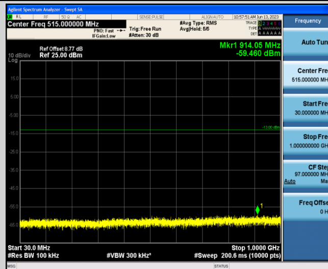
Band4-5MHz-QPSK-19975-1-0-Low-30-1000--59.46-PASS
