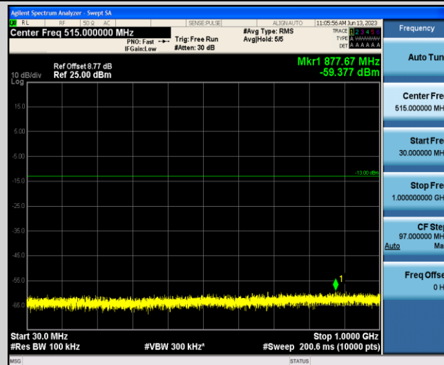
Band4-20MHz-QPSK-20050-1-0-Low-30-1000--59.38-PASS
