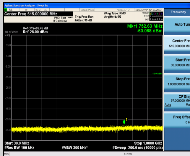
Band4-10MHz-QPSK-20350-1-0-Low-30-1000--60.07-PASS
