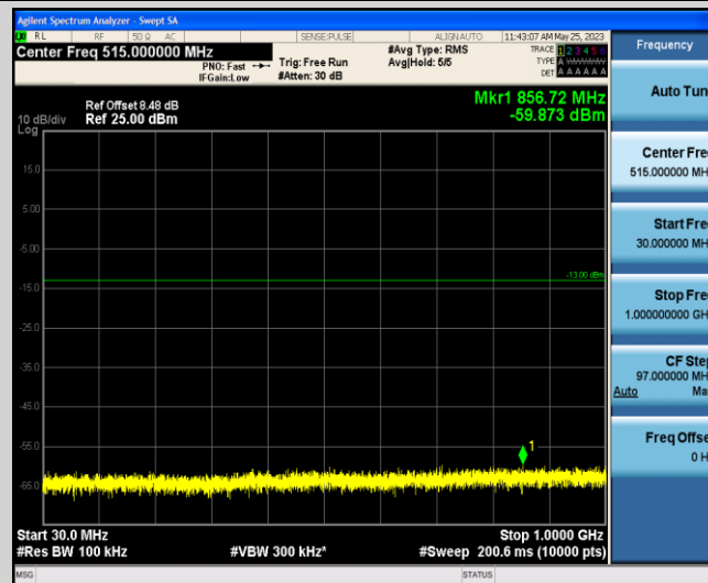
Band66-10MHz-QPSK-132322-1-0-Low-30-1000--59.87-PASS
