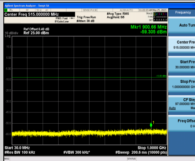
Band66-3MHz-16QAM-132322-1-0-Low-30-1000--59.31-PASS
