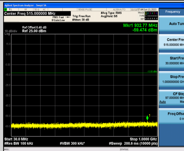
Band66-1.4MHz-QPSK-132665-1-0-Low-30-1000--59.47-PASS
