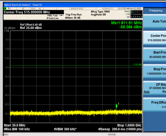
Band66-5MHz-16QAM-132647-1-0-Low-30-1000--59.38-PASS
