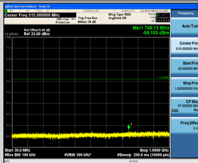
Band66-5MHz-QPSK-132647-1-0-Low-30-1000--59.15-PASS
