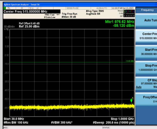
Band66-10MHz-QPSK-132622-1-0-Low-30-1000--59.12-PASS
