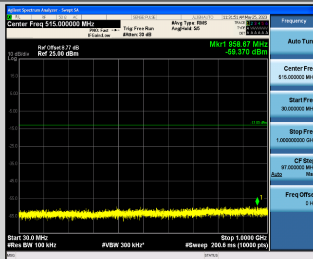
Band66-5MHz-QPSK-131997-1-0-Low-30-1000--59.37-PASS
