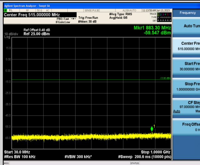
Band66-3MHz-QPSK-132657-1-0-Low-30-1000--59.55-PASS
