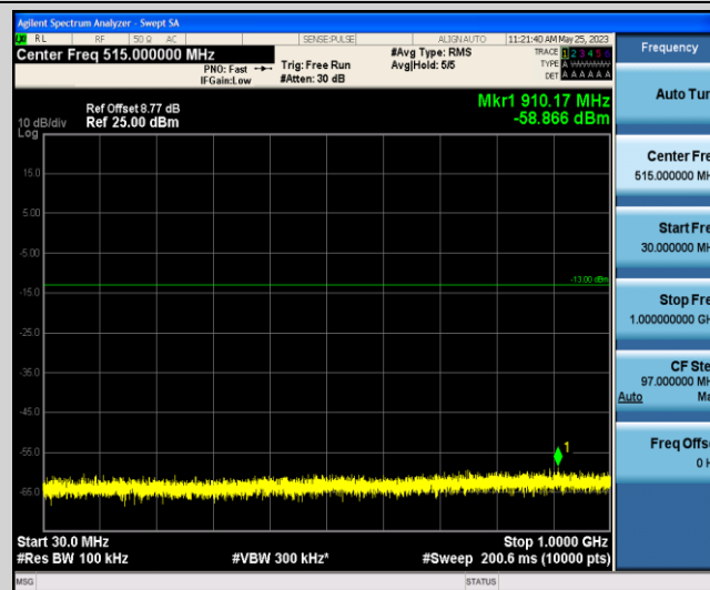
Band66-3MHz-16QAM-131987-1-0-Low-30-1000--58.87-PASS
