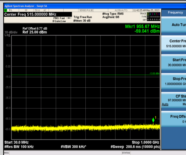
Band66-10MHz-QPSK-132022-1-0-Low-30-1000--59.04-PASS
