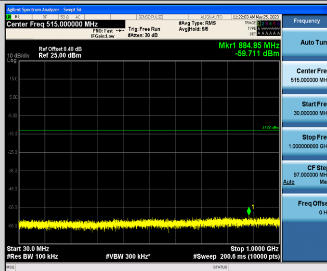
Band66-3MHz-QPSK-132322-1-0-Low-30-1000--59.71-PASS
