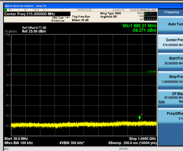
Band66-3MHz-QPSK-131987-1-0-Low-30-1000--59.27-PASS
