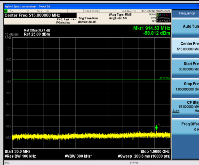
Band66-1.4MHz-QPSK-131979-1-0-Low-30-1000--58.81-PASS
