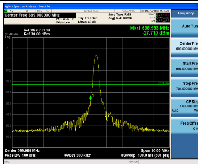
Band12-5MHz-QPSK-23035-1-0-Low--27.71-PASS
