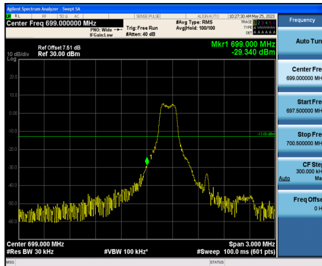
Band12-1.4MHz-QPSK-23017-1-0-Low--29.34-PASS
