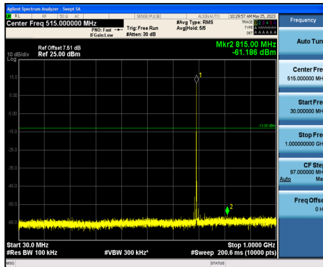
Band12-1.4MHz-QPSK-23017-1-0-Low-30-1000--61.19-PASS
