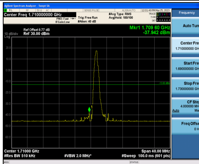
Band66-20MHz-16QAM-132072-1-0-Low--37.94-PASS
