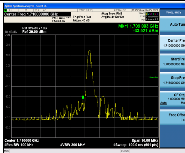
Band66-5MHz-QPSK-131997-1-0-Low--33.52-PASS
