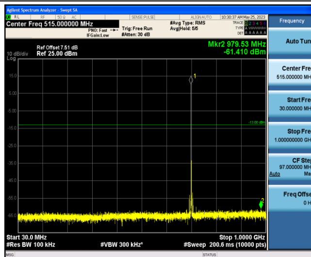
Band12-1.4MHz-QPSK-23095-1-0-Low-30-1000--61.41-PASS
