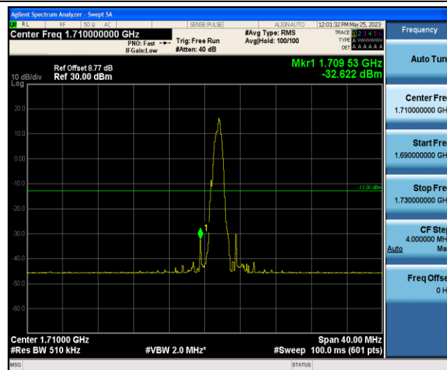
Band66-20MHz-QPSK-132072-1-0-Low--32.62-PASS
