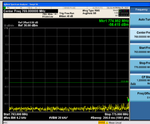
Band13-5MHz-QPSK-23230-1-0-Low-763-775--58.42-PASS
