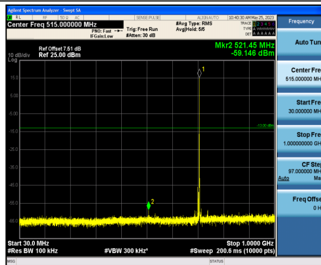
Band12-3MHz-16QAM-23165-1-0-Low-30-1000--59.15-PASS
