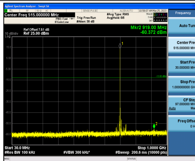
Band12-10MHz-QPSK-23130-1-0-Low-30-1000--60.37-PASS
