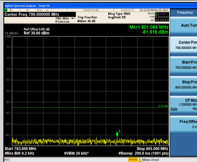
Band13-5MHz-QPSK-23230-1-0-Low-793-805--61.92-PASS
