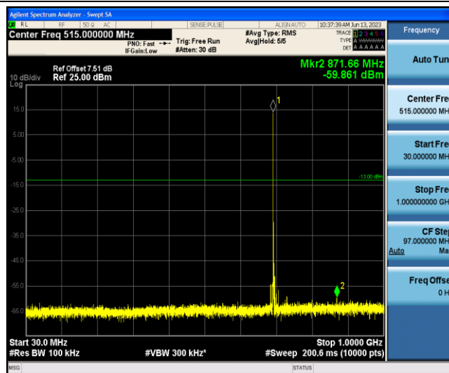
Band12-10MHz-QPSK-23060-1-0-Low-30-1000--59.86-PASS
