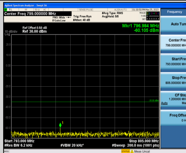
Band13-5MHz-QPSK-23205-1-0-Low-793-805--60.11-PASS
