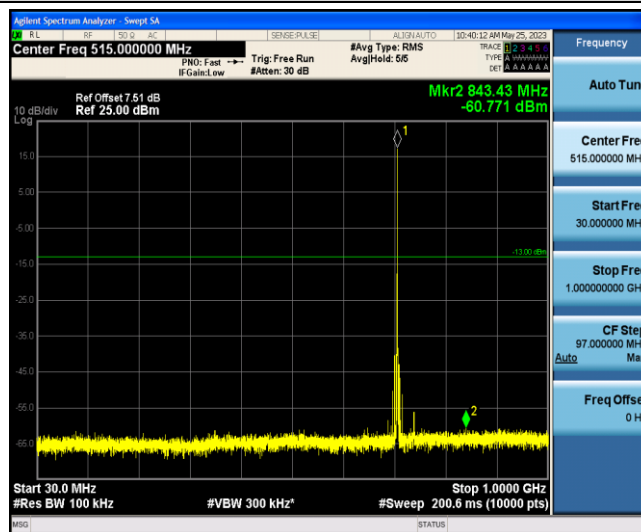
Band12-3MHz-QPSK-23165-1-0-Low-30-1000--60.77-PASS
