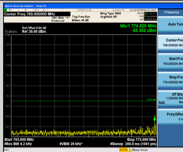
Band13-5MHz-QPSK-23205-1-0-Low-763-775--55.35-PASS
