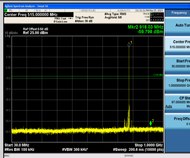
Band13-5MHz-QPSK-23230-1-0-Low-30-1000--59.8-PASS
