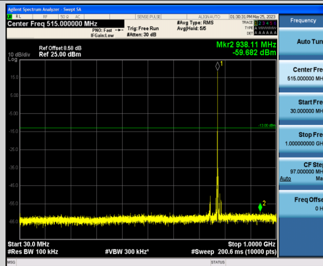
Band13-5MHz-QPSK-23205-1-0-Low-30-1000--59.68-PASS
