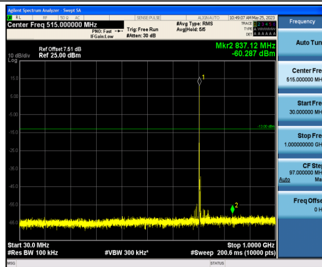
Band12-5MHz-QPSK-23155-1-0-Low-30-1000--60.29-PASS
