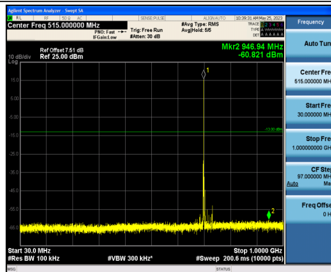
Band12-3MHz-QPSK-23095-1-0-Low-30-1000--60.82-PASS
