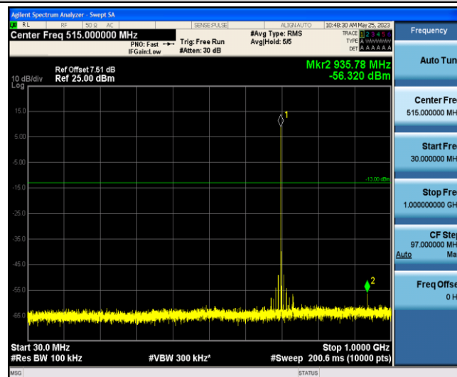
Band12-5MHz-QPSK-23095-1-0-Low-30-1000--56.32-PASS
