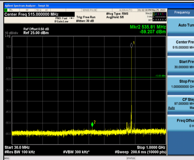
Band13-5MHz-QPSK-23255-1-0-Low-30-1000--59.21-PASS
