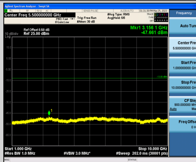
Band13-5MHz-QPSK-23230-1-0-Low-1000-10000--47.66-PASS
