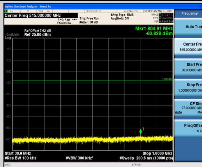
Band2-3MHz-QPSK-18900-1-0-Low-30-1000--60.83-PASS
