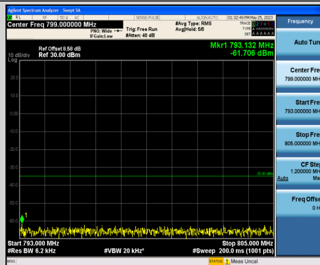
Band13-5MHz-QPSK-23255-1-0-Low-793-805--61.71-PASS
