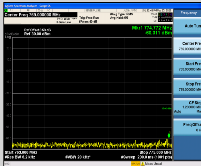
Band13-5MHz-QPSK-23255-1-0-Low-763-775--60.31-PASS
