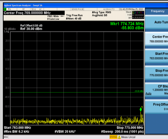
Band13-10MHz-QPSK-23230-1-0-Low-763-775--55.8-PASS
