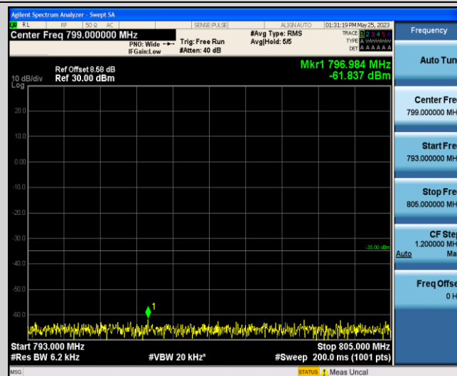
Band13-5MHz-16QAM-23205-1-0-Low-793-805--61.84-PASS
