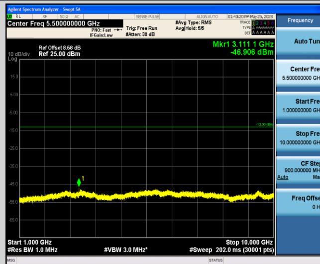
Band13-10MHz-QPSK-23230-1-0-Low-1000-10000--46.91-PASS
