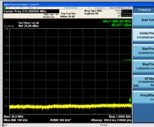
Band2-5MHz-QPSK-19175-1-0-Low-30-1000--60.98-PASS
