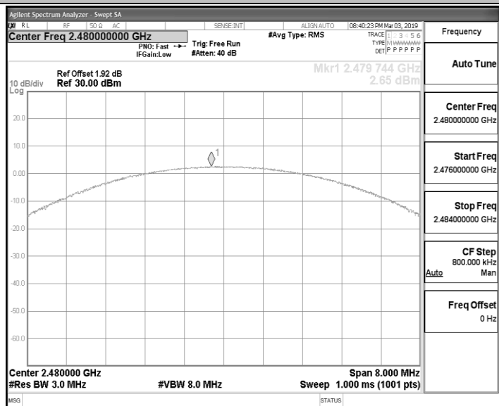
3DH1_Ant1_2480
