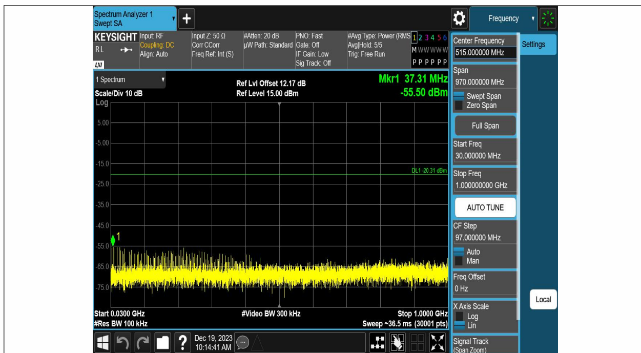
BLE_2M-Ant1-2480-30~1000-PASS
