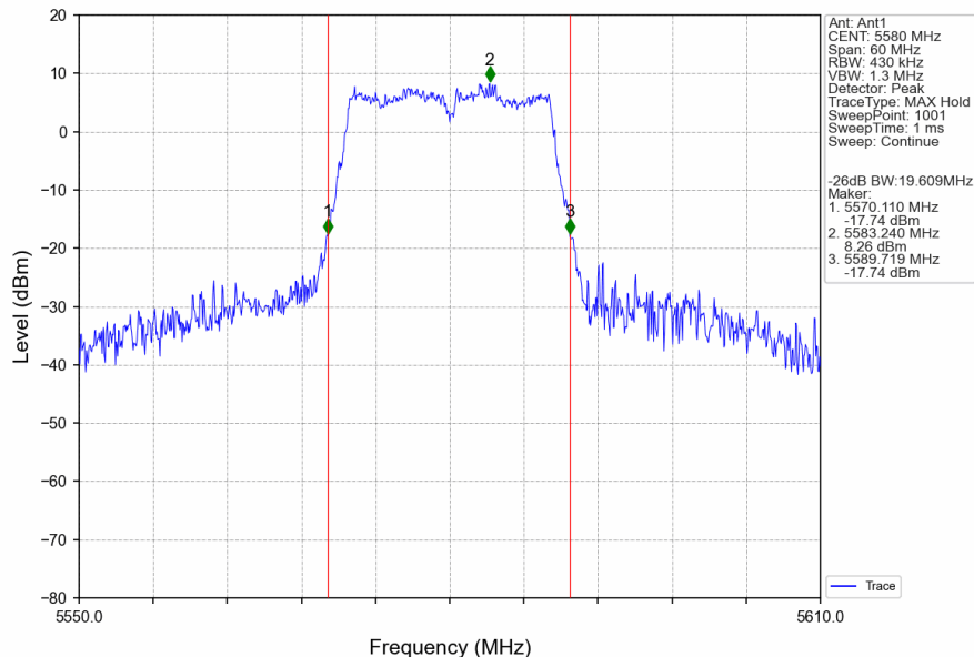
802.11a_MCH_5580MHz_Ant1_NTNV
