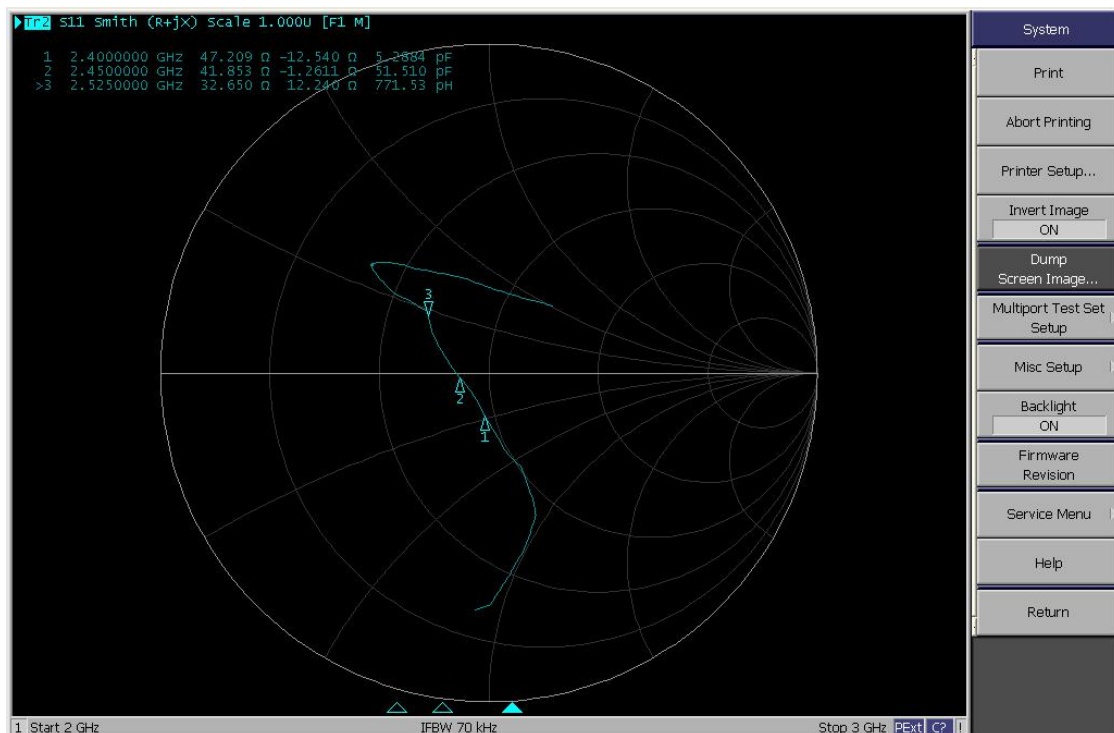
Smith 图
