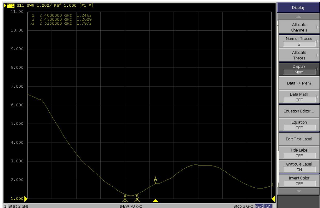
驻波图
