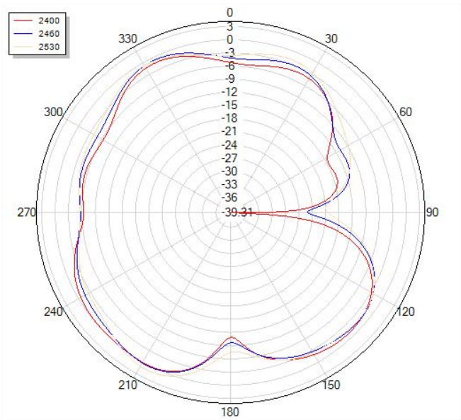
Phi=90
