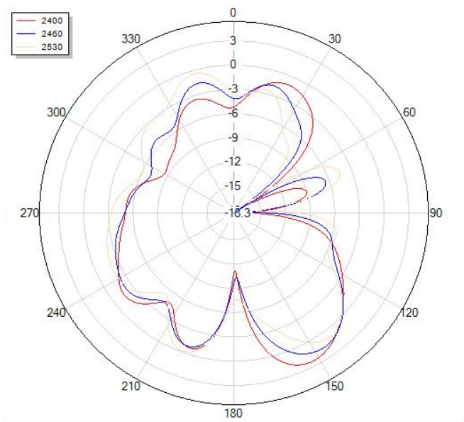
Theta=90
