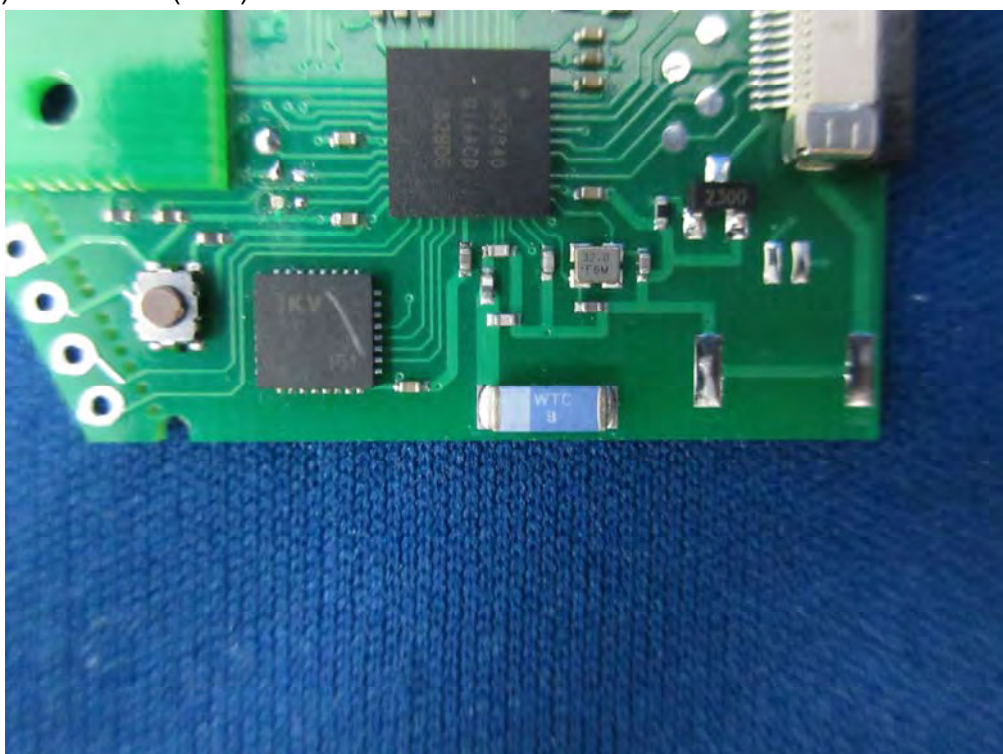
(27) EUT Photo (ANT)
