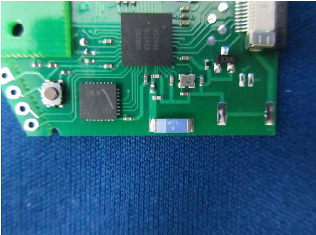
(12) EUT Photo (M/N: W20)
