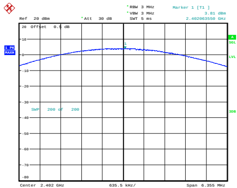
\pi/4 -DQPSK_Low 3.81dBm
