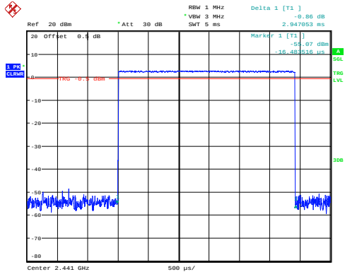
GFSK_Hopping_DH5 2.947ms
