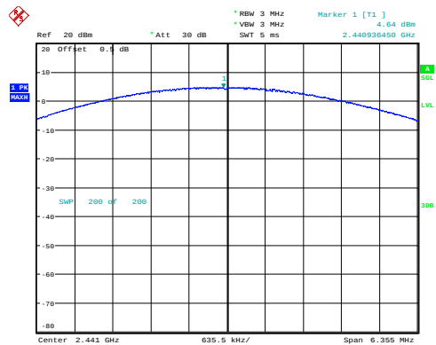
\pi/4 -DQPSK_Middle 4.64dBm
