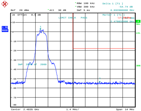
\pi/4 -DQPSK_High 54.74dB
