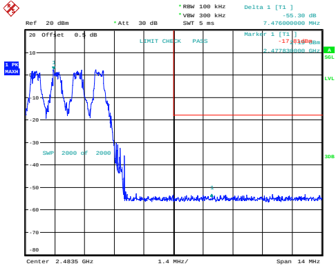
GFSK_Hopping_Upper 55.30dB
