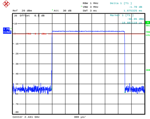
GFSK_Hopping_DH3 1.675ms
