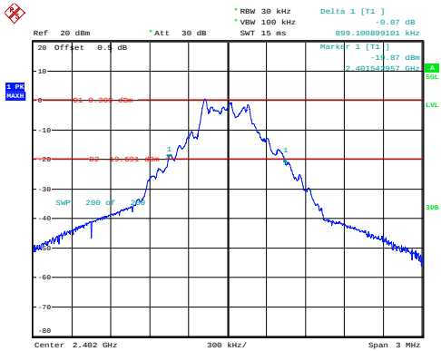
GFSK_Low 0.899MHz
