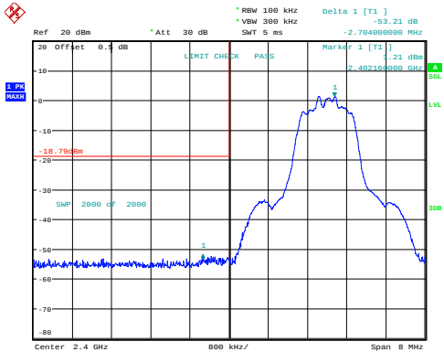
\pi/4 -DQPSK_Low 53.21dB
