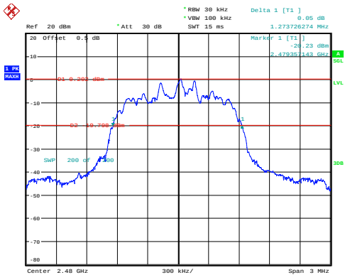
\pi/4 -DQPSK_High 1.274MHz
