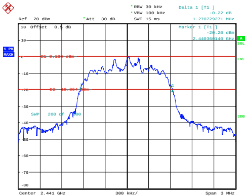
\pi/4 -DQPSK_Middle 1.271MHz
