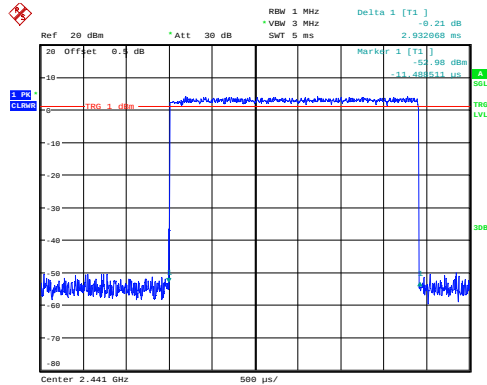
\pi/4 -DQPSK_Hopping_2DH5 2.932ms
