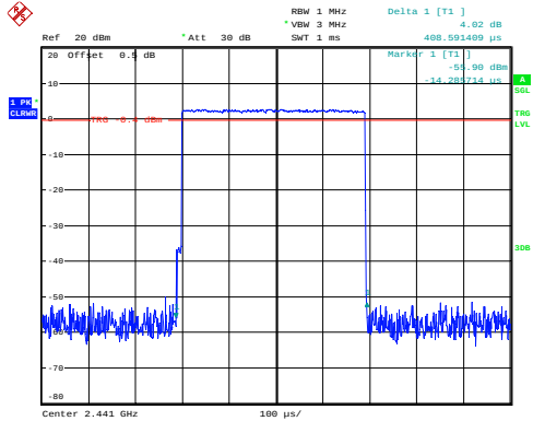
GFSK_Hopping_DH1 0.409ms
