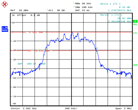
\pi/4 -DQPSK_Low 1.271MHz
