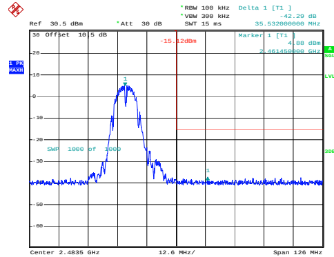
802.11b_2462MHz
