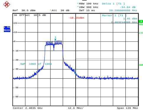
802.11n20_2462MHz
