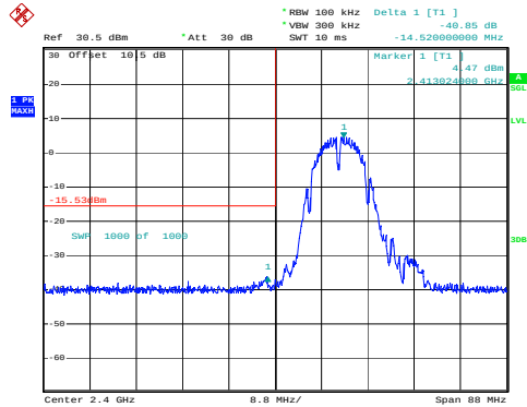
802.11b_2412MHz
