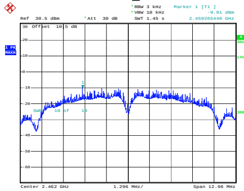
802.11b_2462MHz
