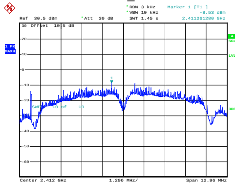
802.11b_2412MHz
