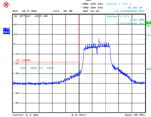
802.11n20_2412MHz
