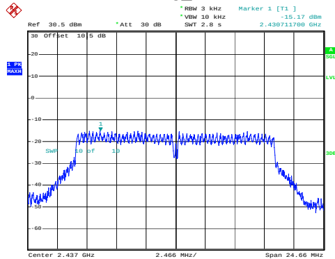
802.11g_2437MHz
