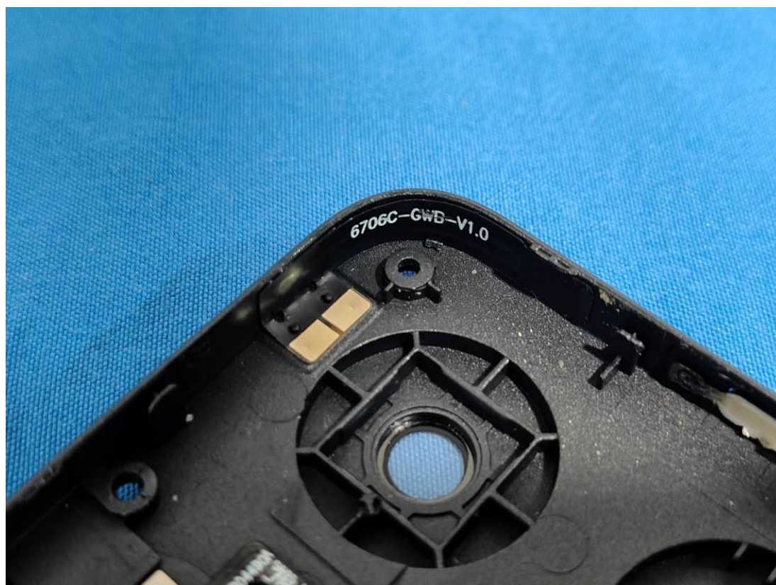
GNSS&Wi-Fi&Bluetooth Antenna
