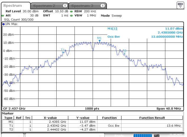
802.11b_2437MHz
