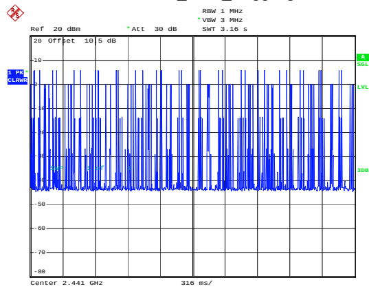
3EDR_DH1_Hopping
