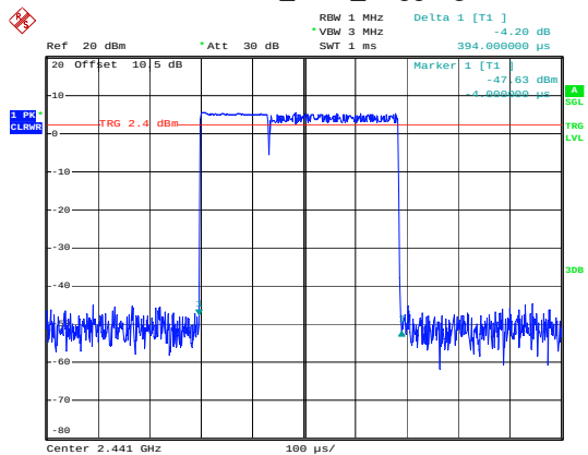
2EDR_DH1_Hopping
