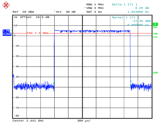
2EDR_DH3_Hopping
