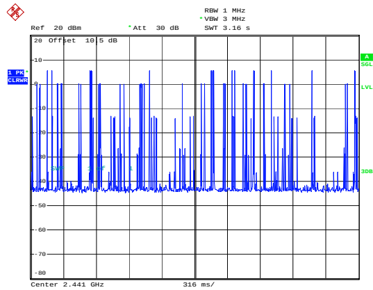
2EDR_DH3_Hopping
