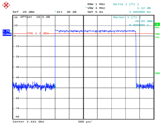
2EDR_DH5_Hopping
