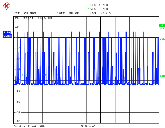
2EDR_DH1_Hopping
