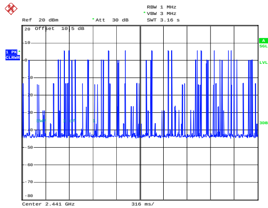
2EDR_DH5_Hopping
