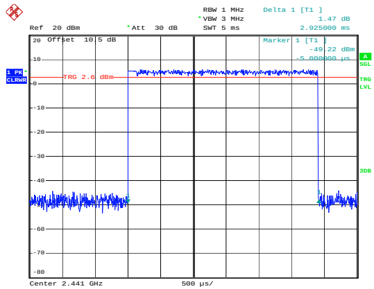
3EDR_DH5_Hopping
