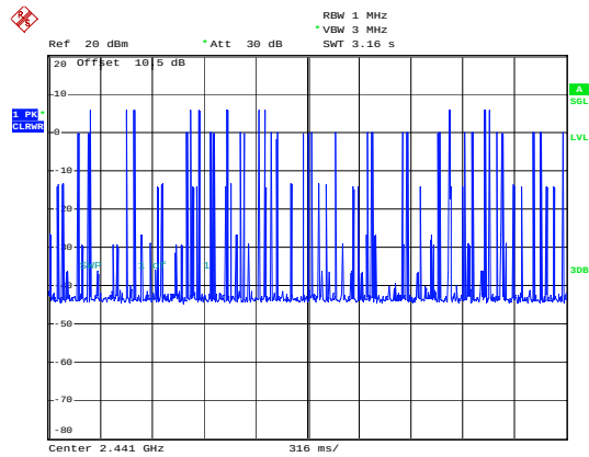
3EDR_DH5_Hopping
