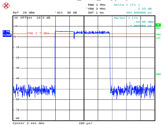
3EDR_DH1_Hopping
