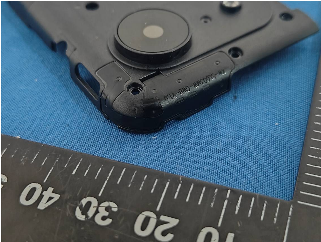
4G DIV Antenna
