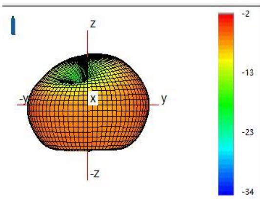
ZX-Plane Total
