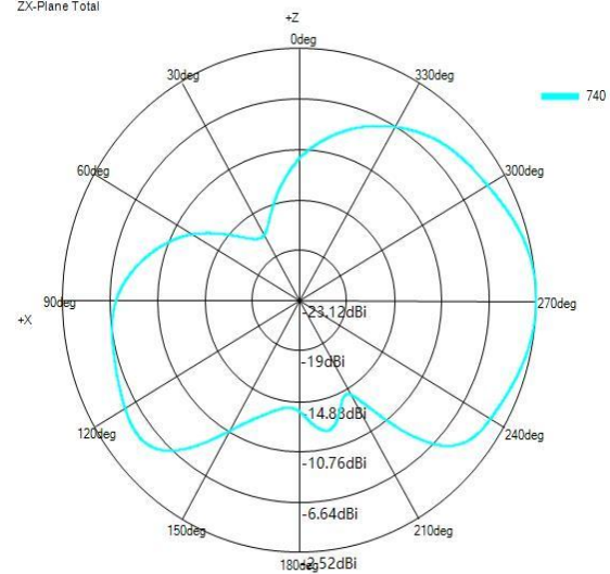
ZX-Plane Total
