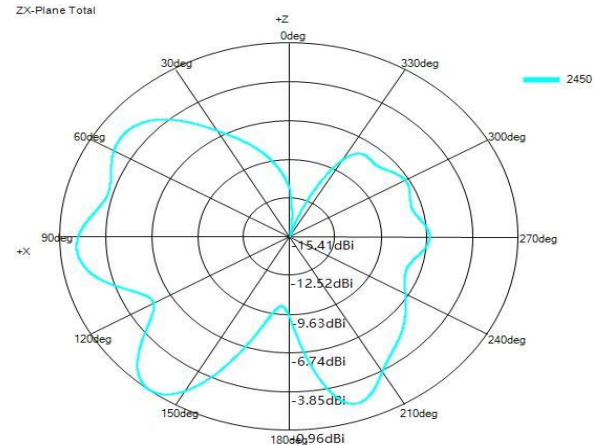
ZX-Plane Total
