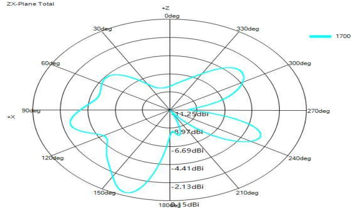
ZX-Plane Total
