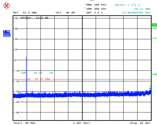
802.11n20_2412MHz
