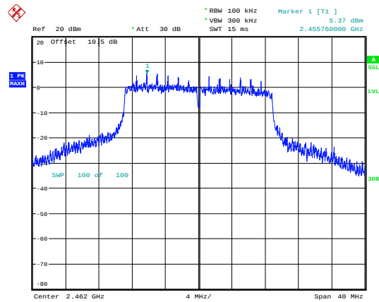
802.11n20_2462MHz
