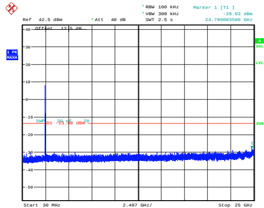
802.11b_2462MHz
