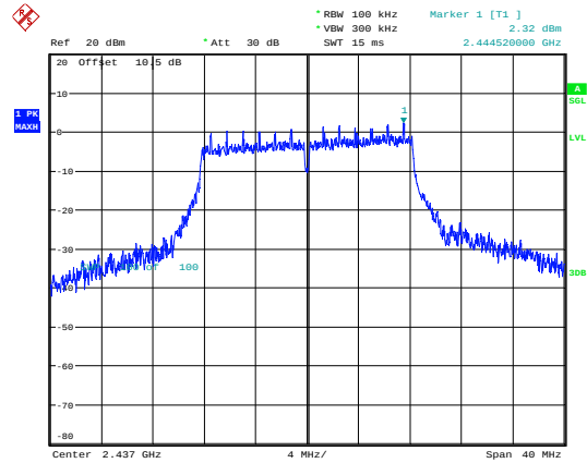
802.11g_2437MHz
