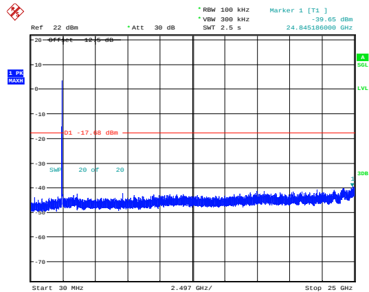
802.11g_2437MHz
