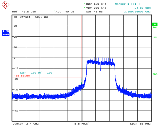
802.11n20_2412MHz
