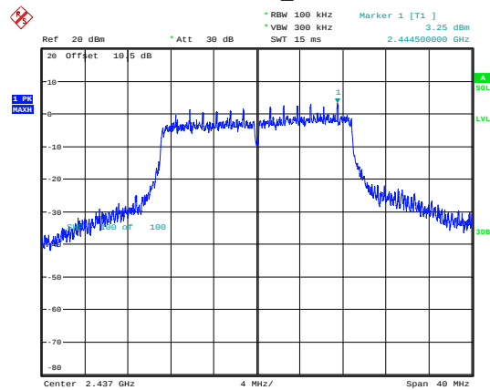
802.11n20_2437MHz
