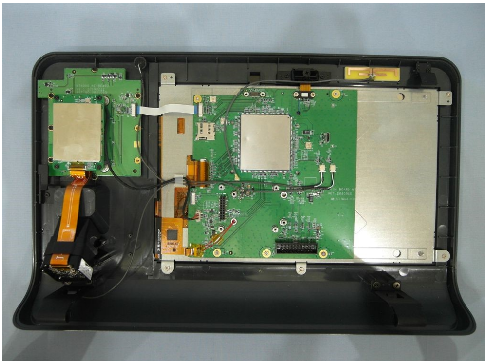
(10) EUT Photo
