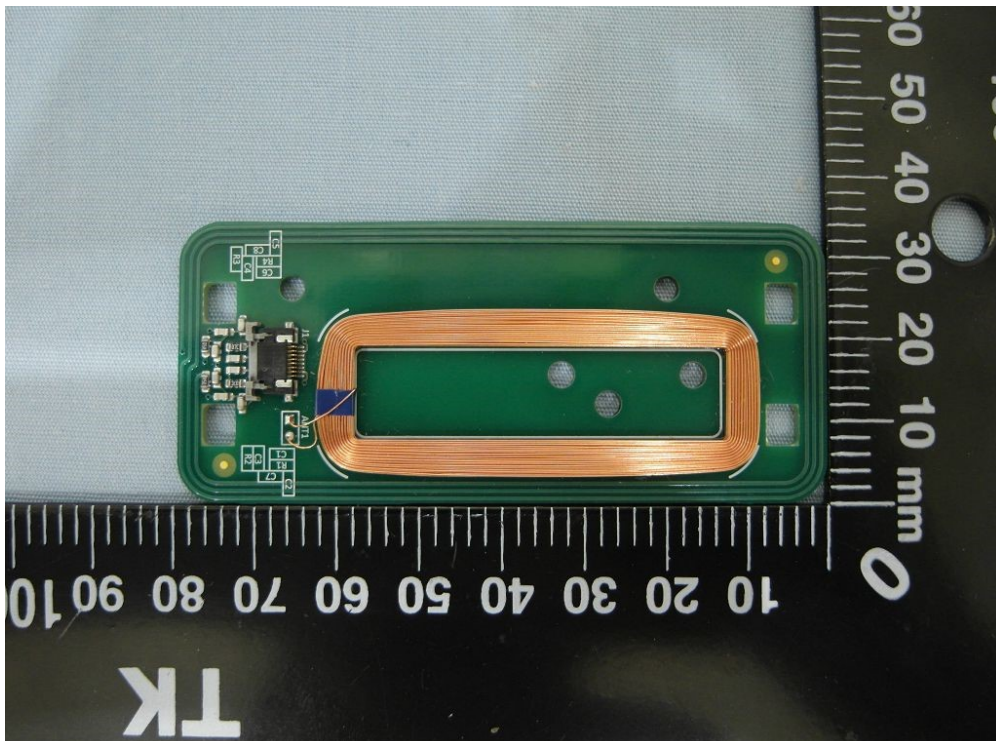
(8) EUT Photo
