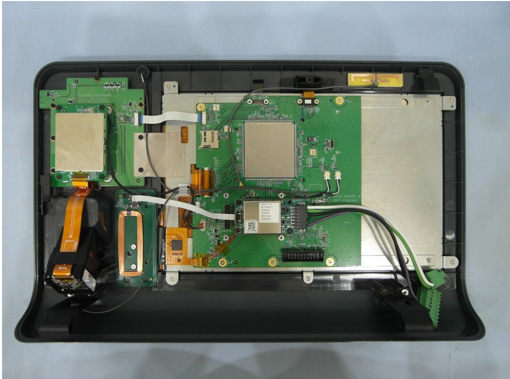
(2) EUT Photo
