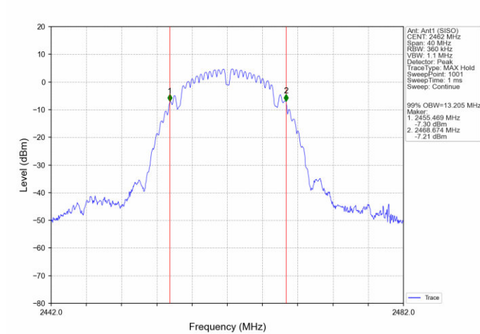
802.11b_HCH_2462MHz_Ant1 (SISO)_NTNV
