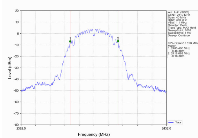
802.11b_LCH_2412MHz_Ant1 (SISO)_NTNV
