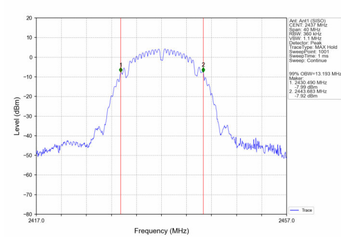
802.11b_MCH_2437MHz_Ant1 (SISO)_NTNV
