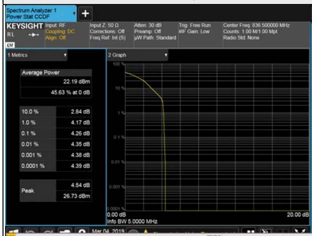
5MHz / 16QAM
