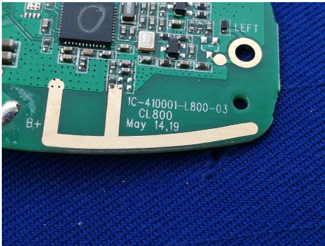
RF ANT
