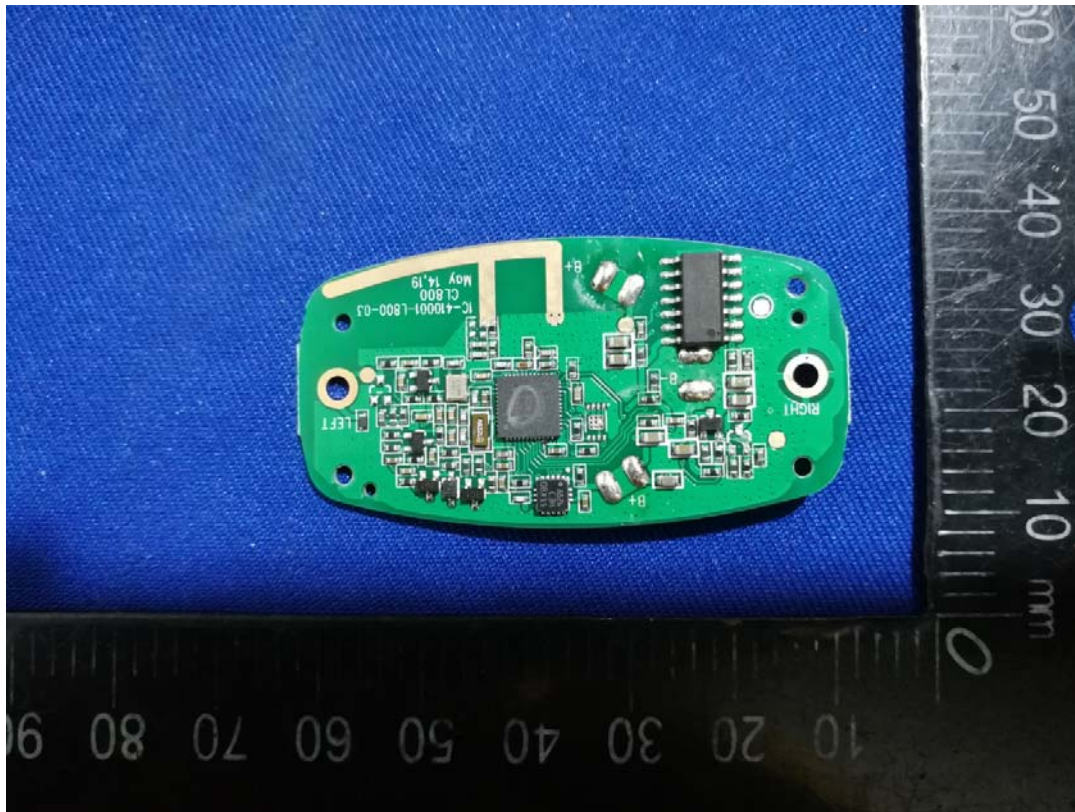
RF ANT
