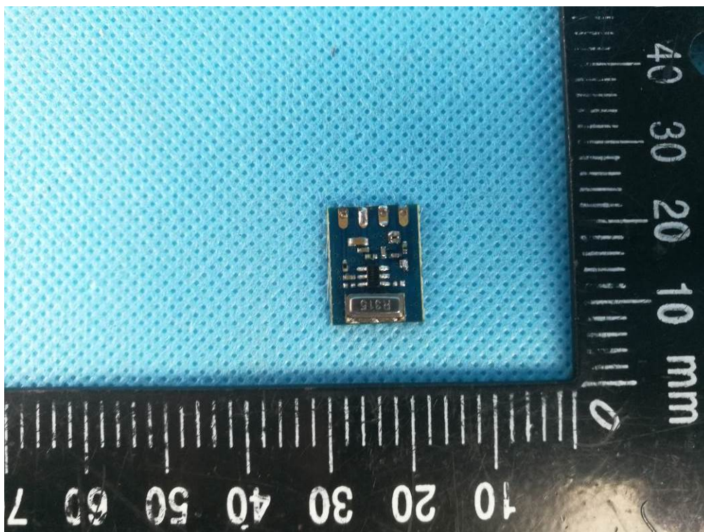
315MHz TX module
