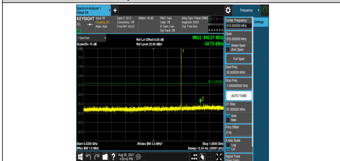
Band12-1.4MHz-QPSK-23095-1-0-Low-30-1000--34.75-PASS
