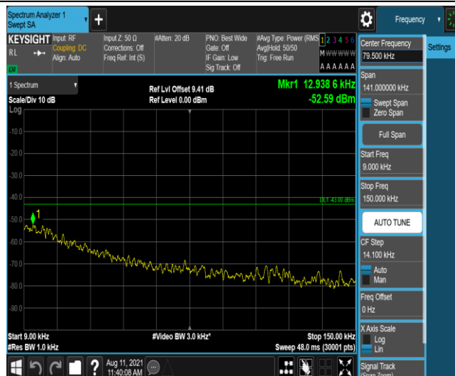
Band25-20MHz-16QAM-26365-1-0-Low-0.009-0.15--52.6-PASS
