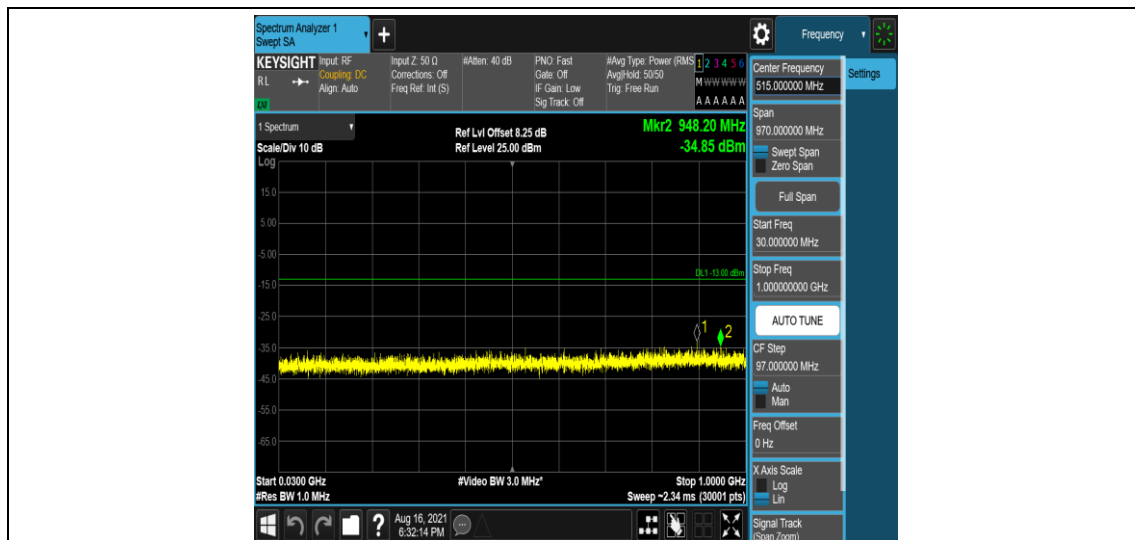
Band26-1.4MHz-QPSK-26740-1-0-Low-30-1000--34.85-PASS
