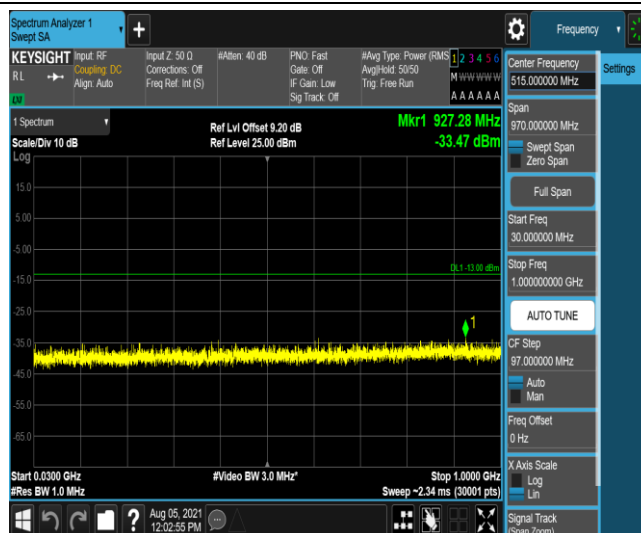
Band4-20MHz-QPSK-20050-1-0-Low-30-1000--33.47-PASS
