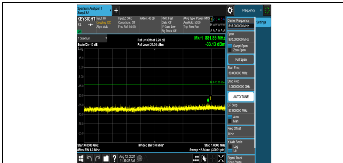
Band66-20MHz-QPSK-132072-1-0-Low-30-1000--33.13-PASS
